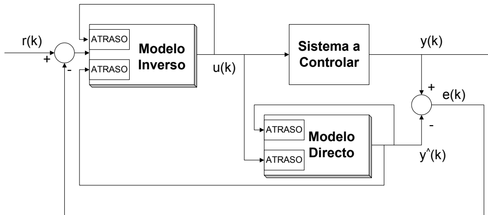
Figura 5.12: Estrutura do IMC com detalhe de implementação dos modelos directo e inverso.
