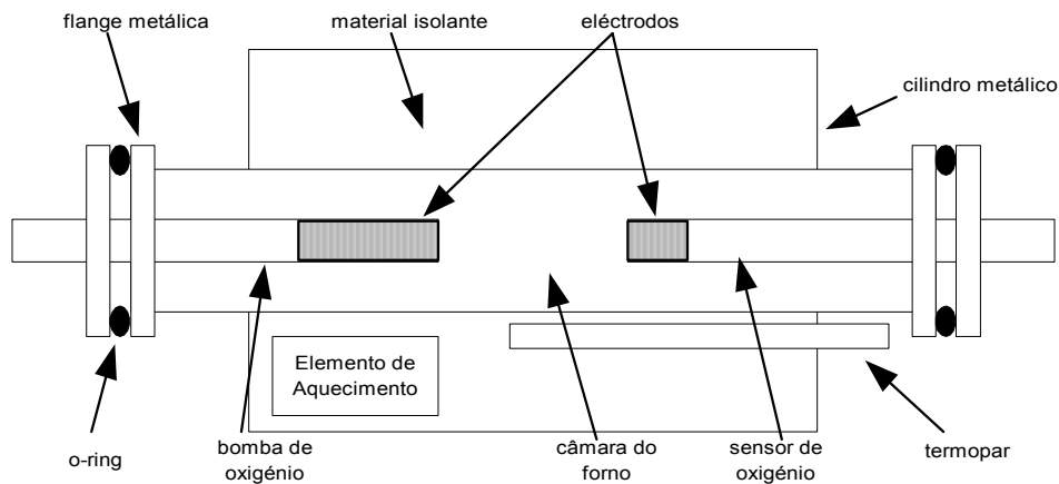
Figura 6.1: Vista esquemática do forno.
