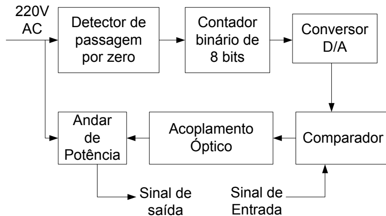
Figura 6.5: Diagrama de blocos do módulo de potência.
