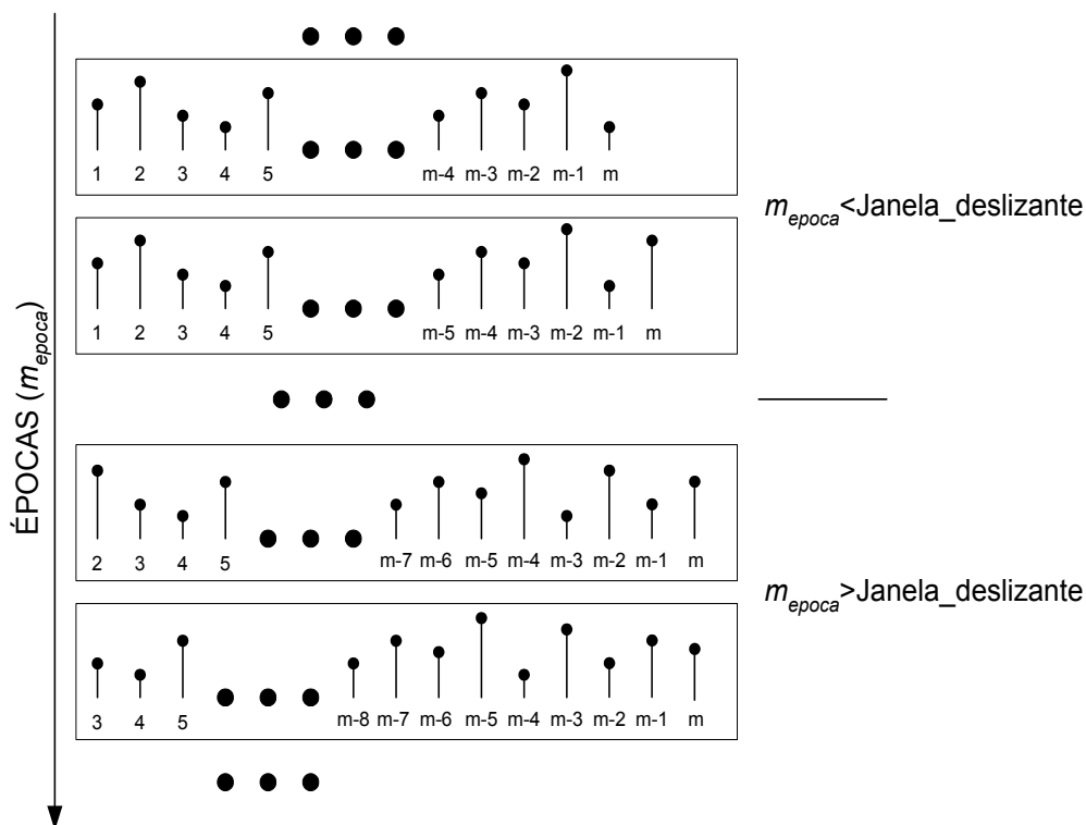
Figura 7.10: Conteúdo da janela deslizante em função da evolução das épocas.
