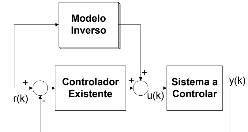
Figura 5.8: Estrutura usada para o Controle Aditivo. Os sinais r(k) , u(k) e y(k) têm o mesmo significado que anteriormente.
