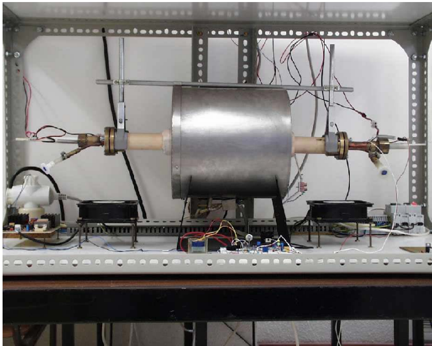
Figura 6.2: Vista exterior do forno.
